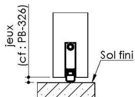
Plinthe automatique
