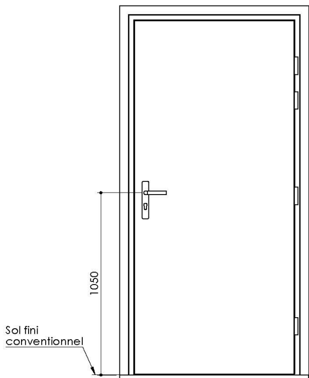
Huisserie isophonique
