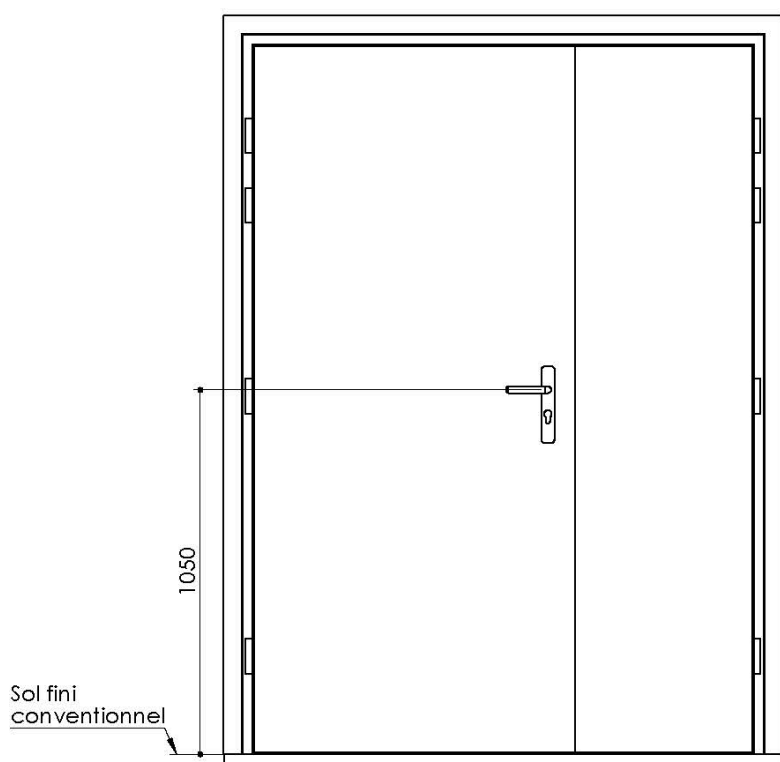
Huisserie isophonique
