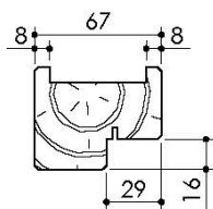
Huisserie isophonique
