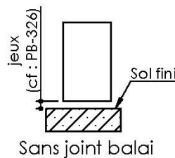
Variantes bas de porte
