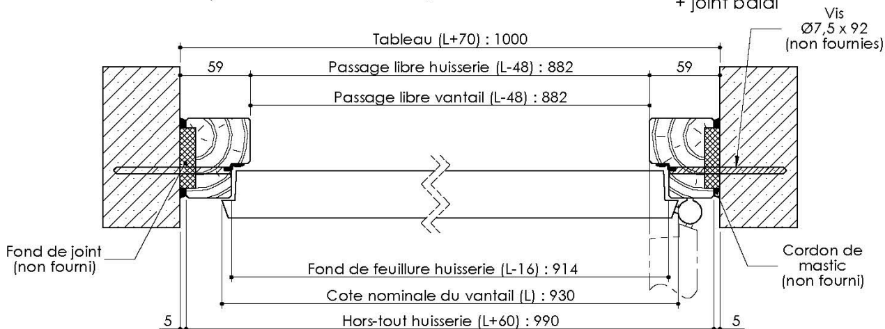
Plinthe automatique
