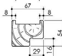
Huisserie isophonique
