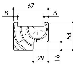
Huisserie isophonique
