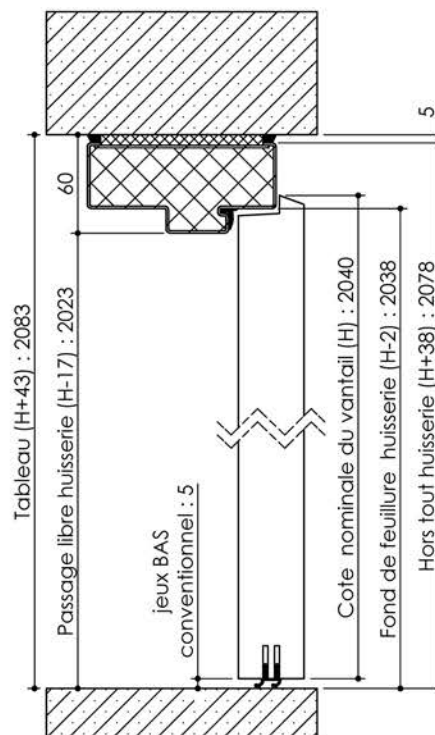
Huisserie isophonique
