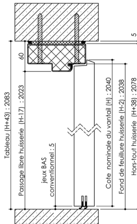
Huisserie isophonique
