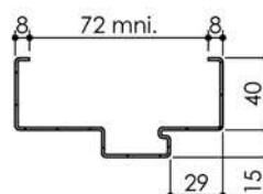
Huisserie isophonique
