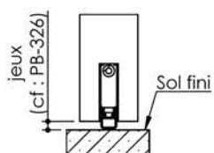
Plinthe automatique
