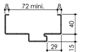
Huisserie isophonique
