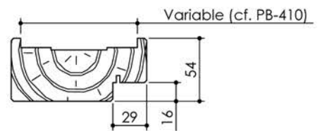
Huisserie isophonique
