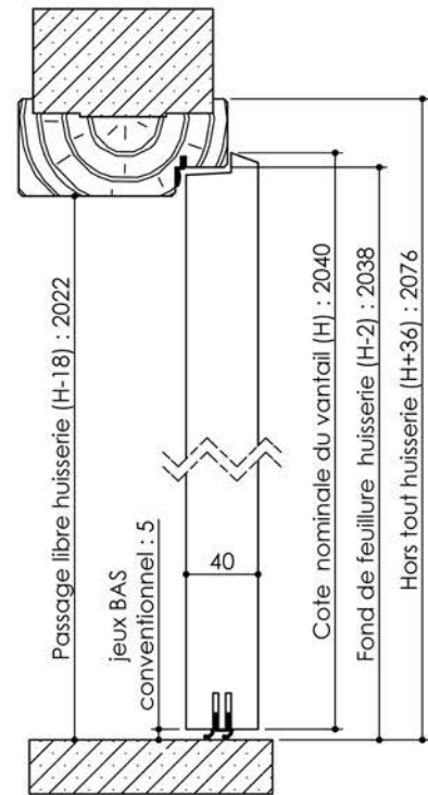
Huisserie isophonique
