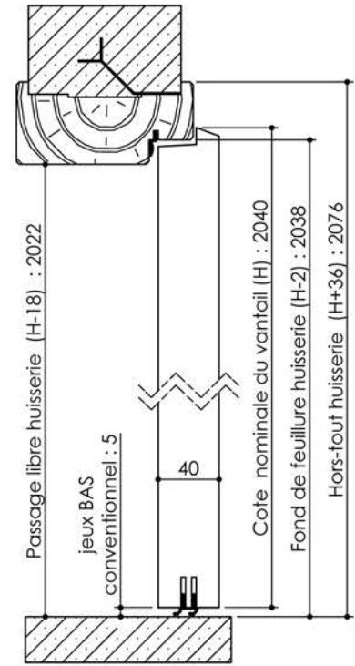
Huisserie isophonique
