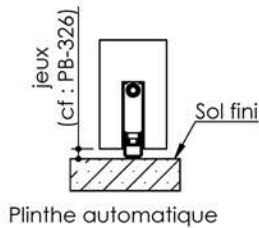
Plinthe automatique
