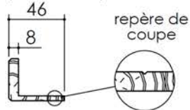
Extension CC S+ cloison 50 à 78 mm (depuis 03/19)
