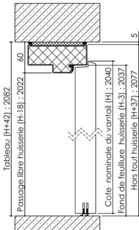
Huisserie isophonique
