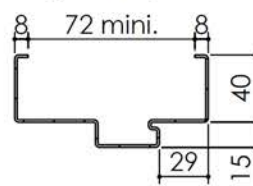
Huisserie isophonique
