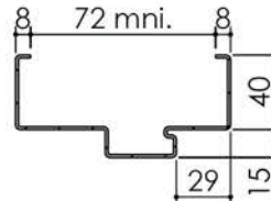
Huisserie isophonique
