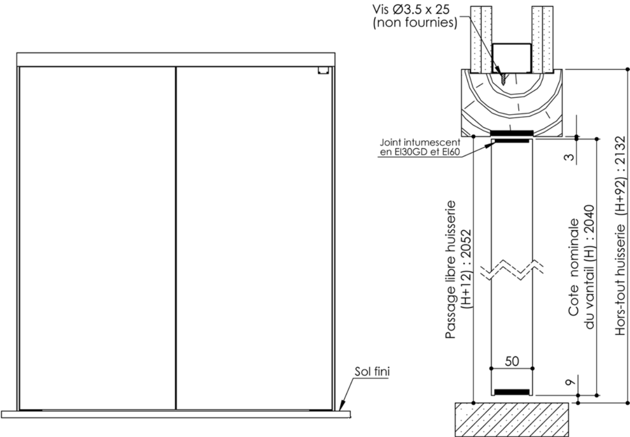
Montant côté articulation
