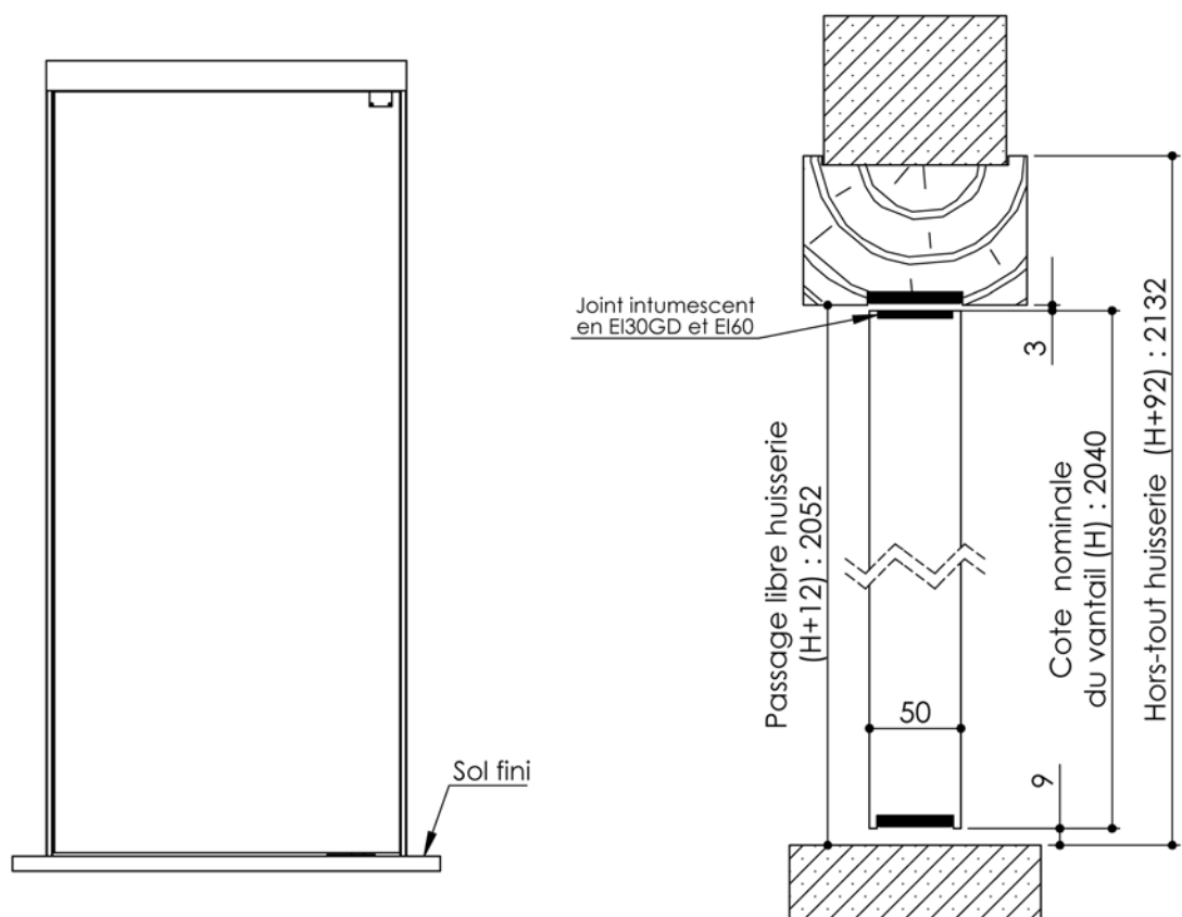
Montant côté battement
