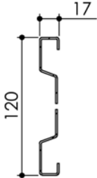
Montant côté articulation
