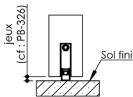
Plinthe automatique
