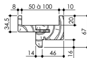
Huisserie isophonique
