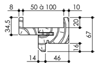
Huisserie isophonique
