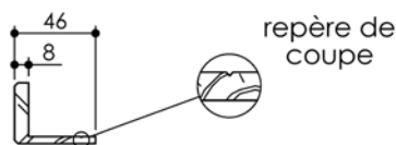
Extension CC S+ cloison 50 à 78 mm (depuis 03/19)
