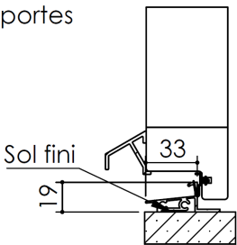
Seuil Alu PMR
