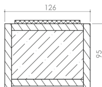
PROFIL MIXTE VV PL EI90 TRAVERSE
