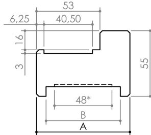
Feuillure 53 x 16 EI 60 Porte à chants droits
