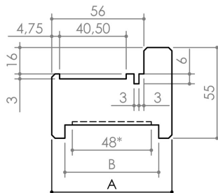
Feuillure ISO 56 x 16 EI 60 Porte à chants droits
