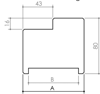
Feuillure 43 x 16 Porte à chants droits Traverse Elargie
