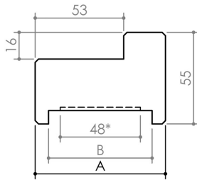
Feuillure 53 x 16 Porte à chants droits
