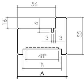
Feuillure ISO 56 x 16 Porte à chants droits
