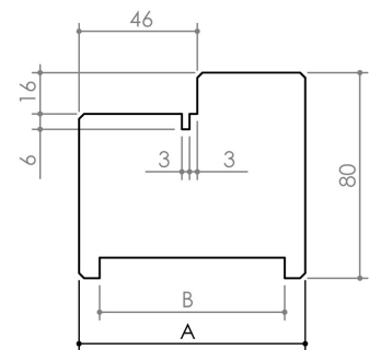
Feuillure ISO 46 x 16 Porte à chants droits Traverse Elargie
