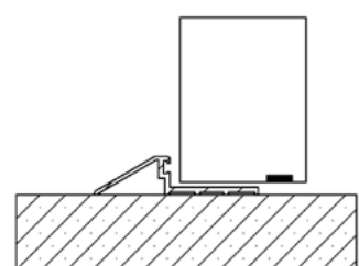
Seuil Alu
