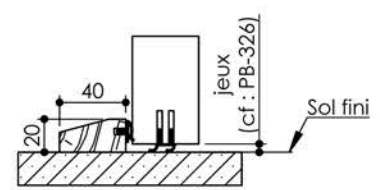
Seuil à la suisse + joint balai
