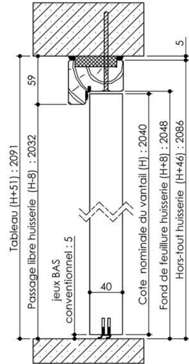
Huisserie isophonique
