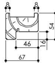
Huisserie isophonique
