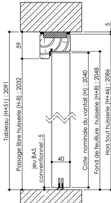
Huisserie isophonique
