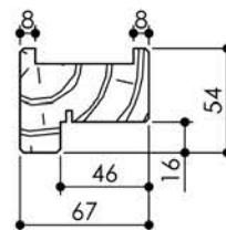
Huisserie isophonique
