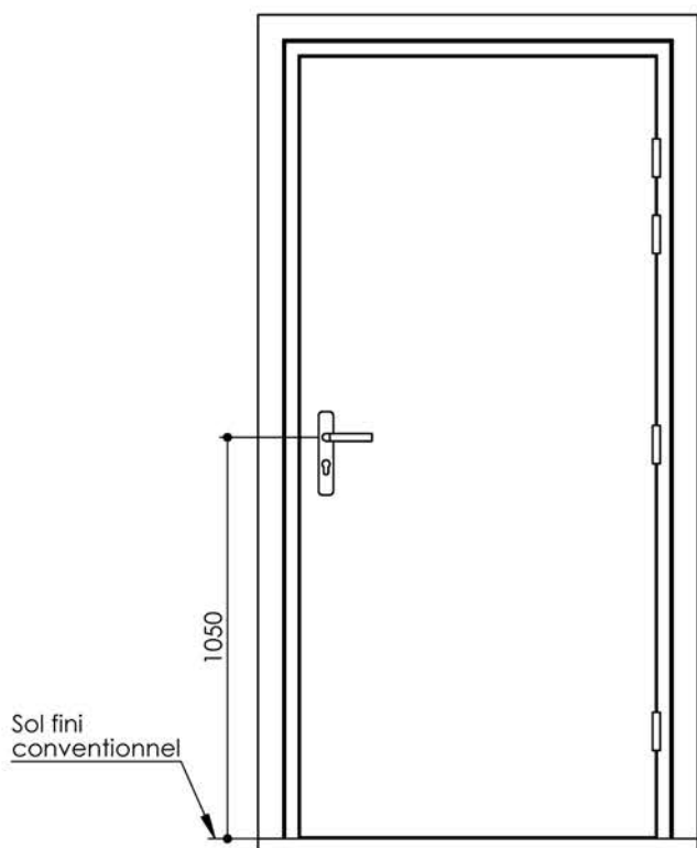
Huisserie non isophonique
