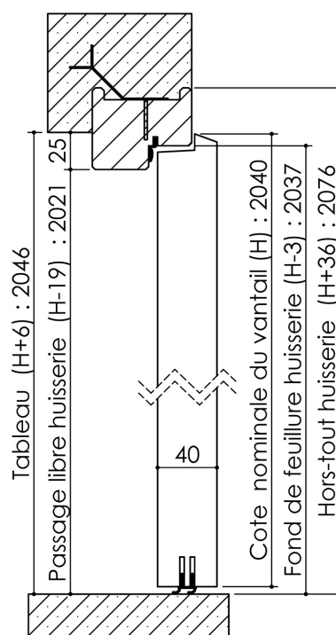
Huisserie isophonique
