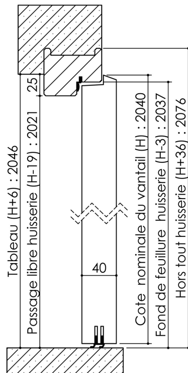
Huisserie isophonique
