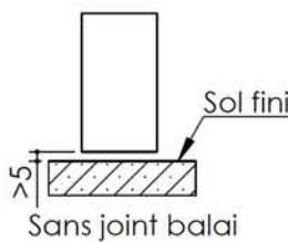
Variantes bas de porte
