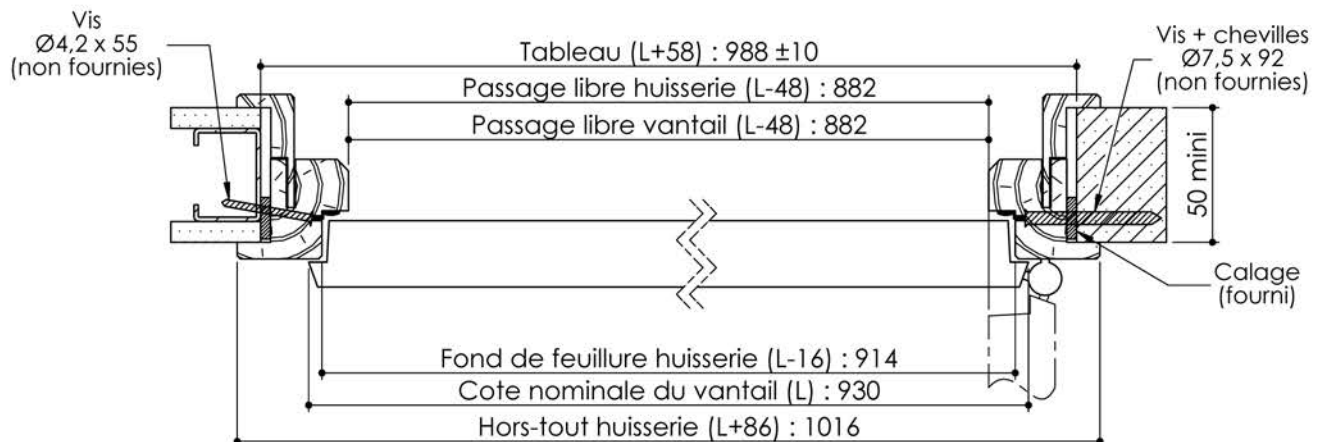
Seuil à la suisse + joint balai
