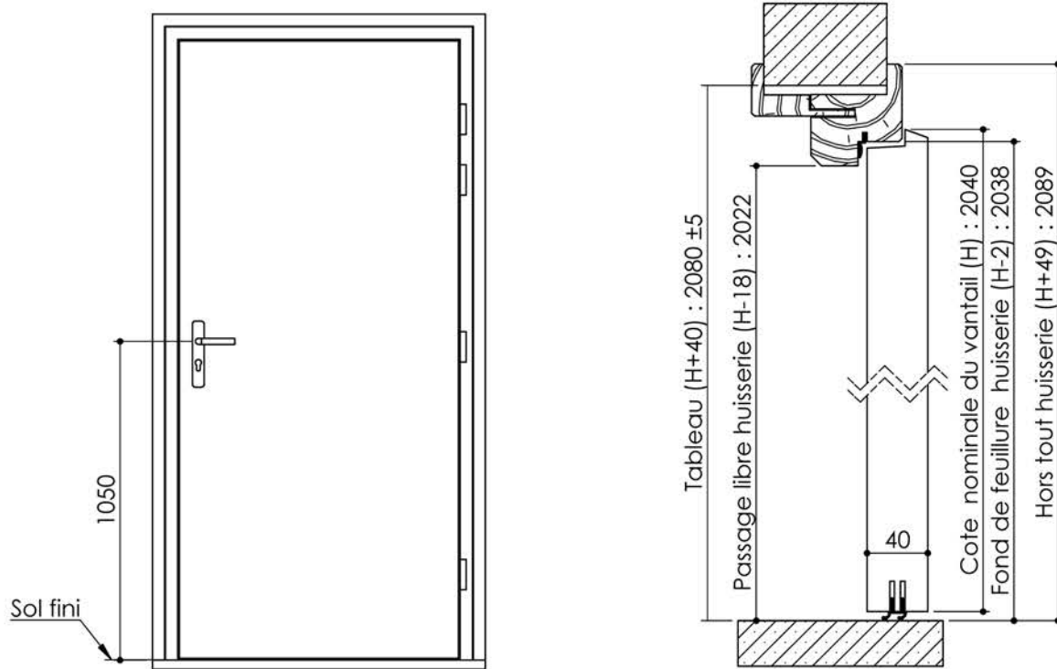
Extension CC S+ cloison 50 à 78 mm (depuis 03/19)
