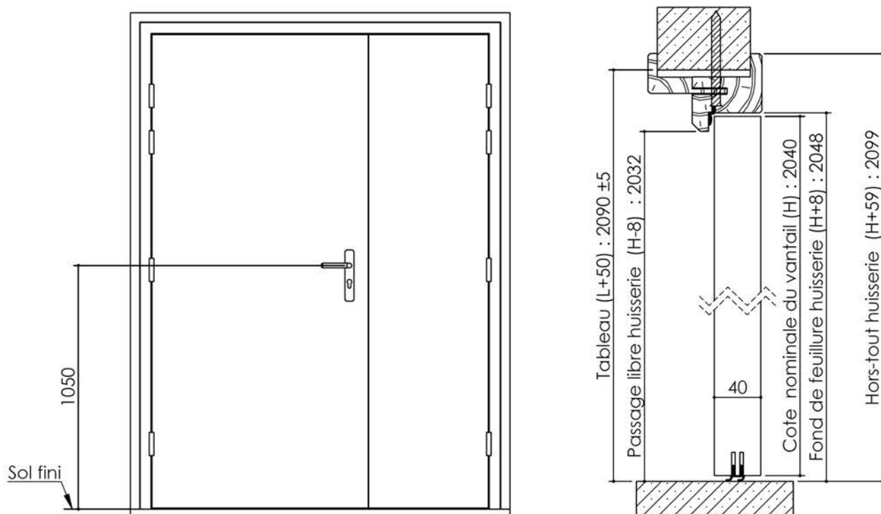
Extension CC S+ cloison 50 à 78 mm (depuis 03/19)
