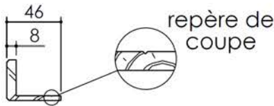
Variantes bas de porte
