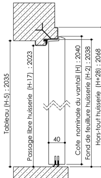
Huisserie isophonique
