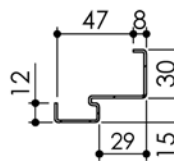
Huisserie isophonique
