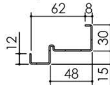
Huisserie isophonique
