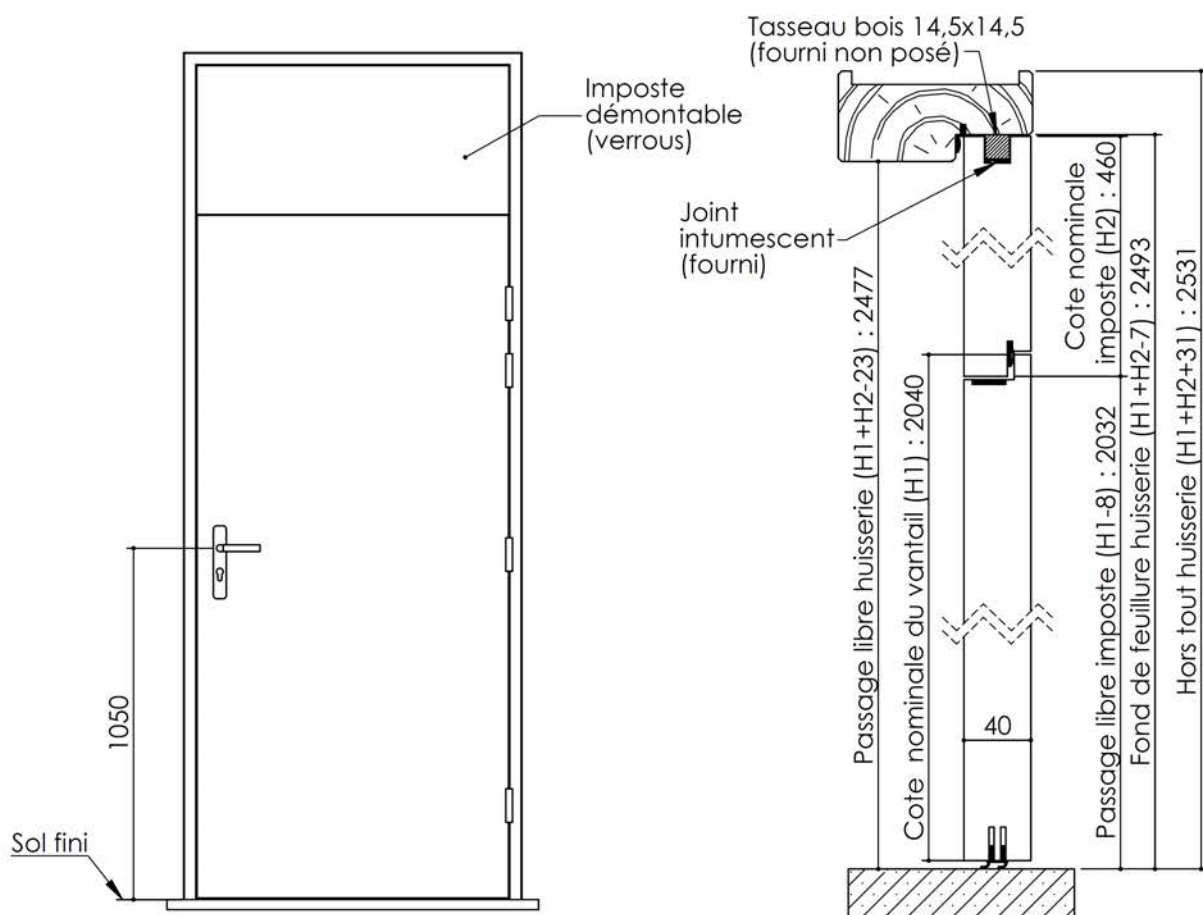
Variante de feuillure imposte
