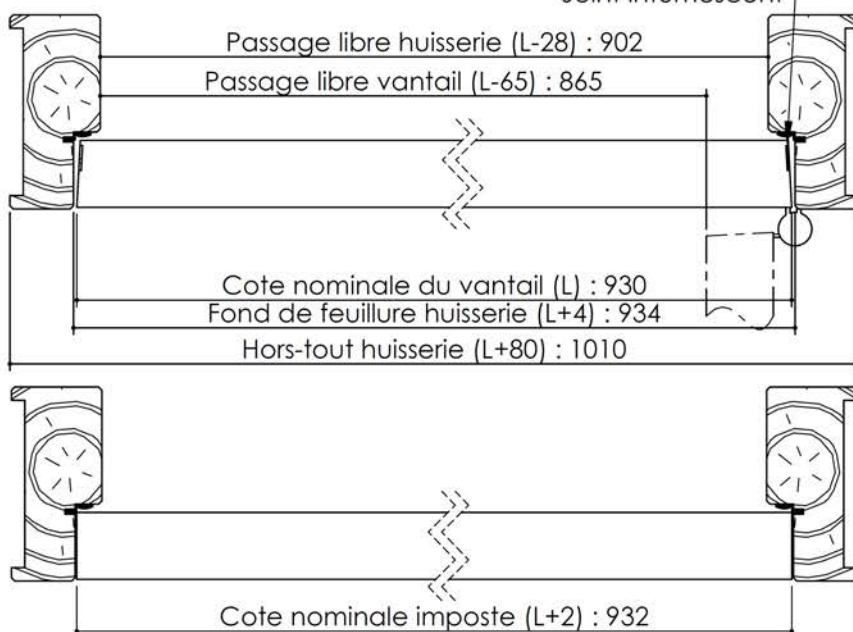
Etanchéité EI300 Joint intumescent
