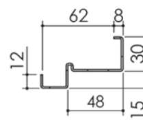
Huisserie isophonique
