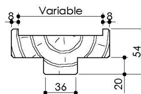
Montant
