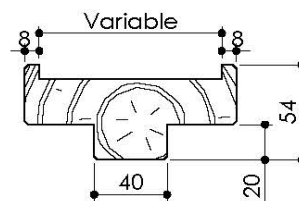
Montant
