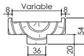
Montant
