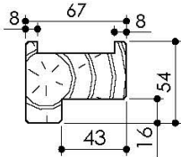
Huisserie non isophonique
