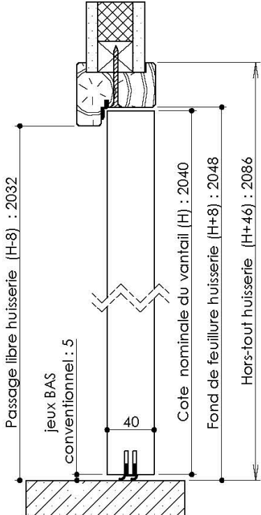
Huisserie non isophonique
