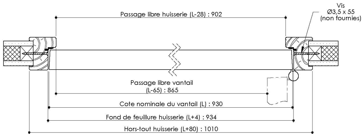
Seuil à la suisse + joint balai
