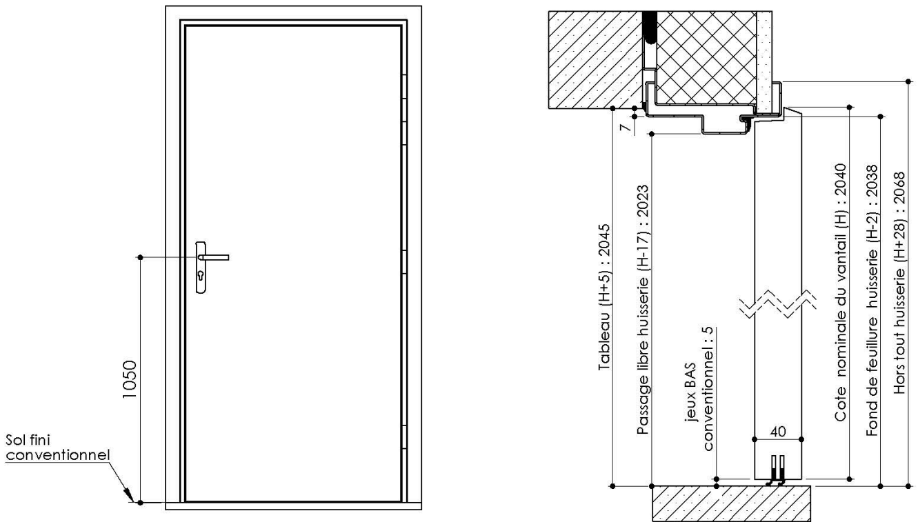
Huisserie isophonique
