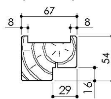
Huisserie isophonique
