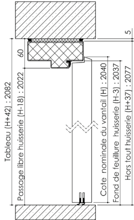
Huisserie isophonique
