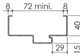
Huisserie isophonique
