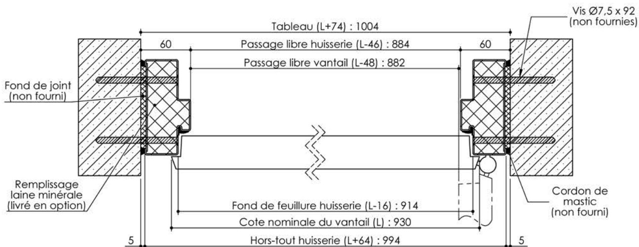
Seuil à la suisse + joint balai
