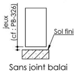
Variantes bas de porte
