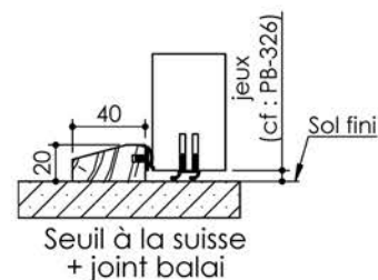
Variantes bas de porte
