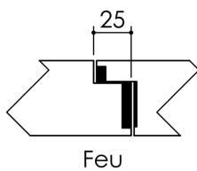
Détail de feuillure centrale de 25
