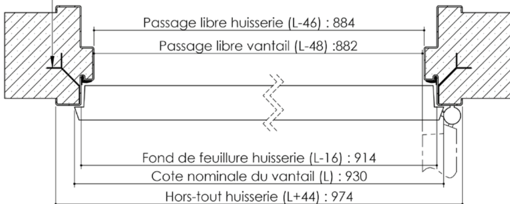
Seuil à la suisse + joint balai
