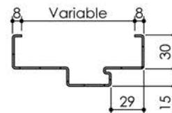
Huisserie isophonique
