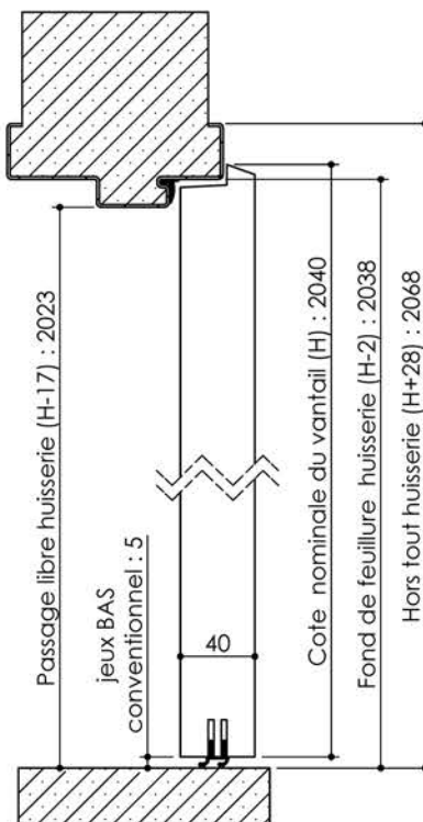
Huisserie isophonique
