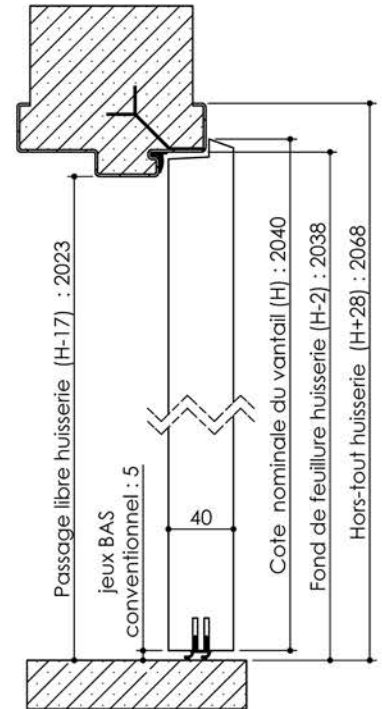
Huisserie isophonique
