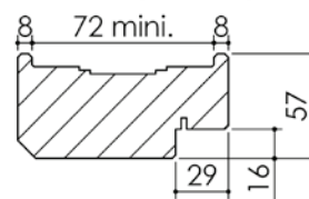
Huisserie isophonique
