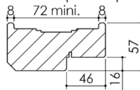
Huisserie isophonique
