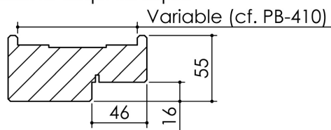
Huisserie isophonique
