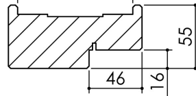
Huisserie isophonique
