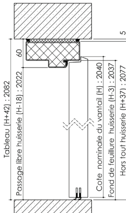
Huisserie isophonique
