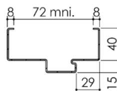
Huisserie isophonique
