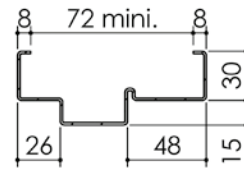
Huisserie isophonique
