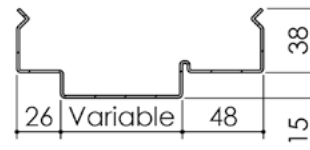
Huisserie isophonique
