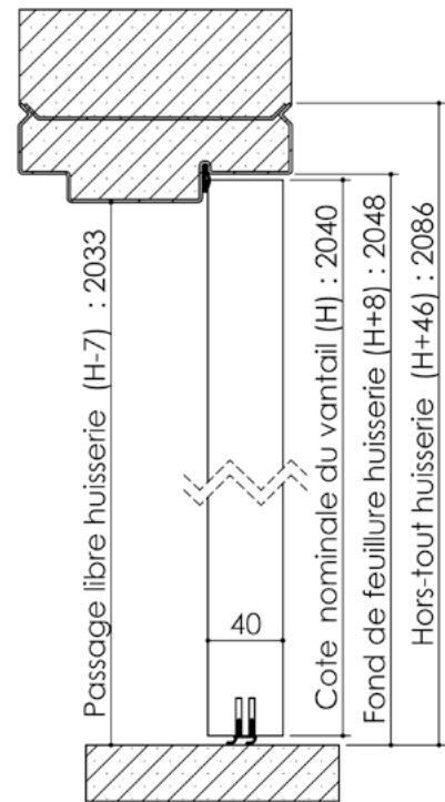
Huisserie isophonique
