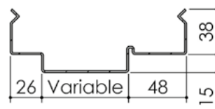
Huisserie isophonique
