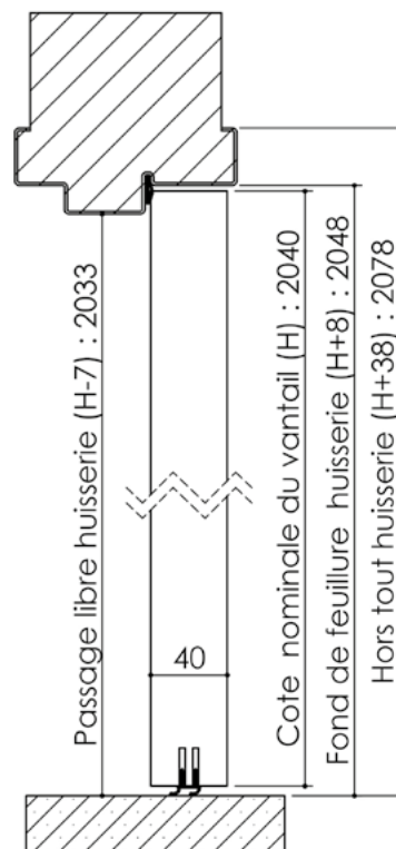
Huisserie isophonique
