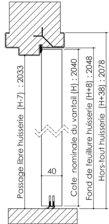
Huisserie isophonique
