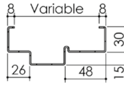
Huisserie isophonique
