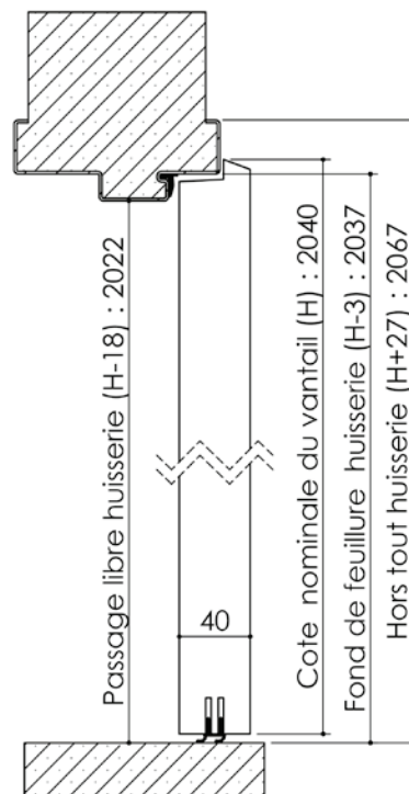
Huisserie isophonique
