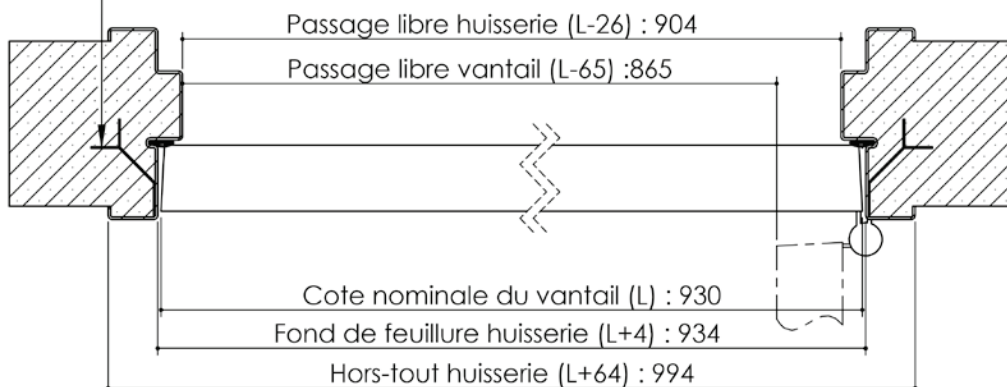
Pattes soudées
