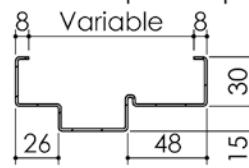
Huisserie isophonique
