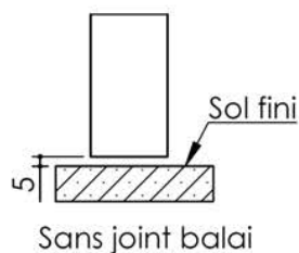
Détail bas de porte
