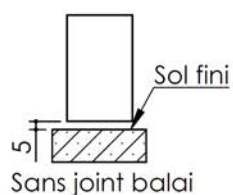
Détail bas de porte
