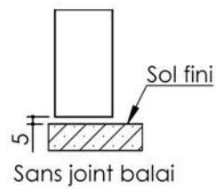
Détail bas de porte
