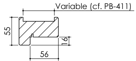
Huisserie isophonique
