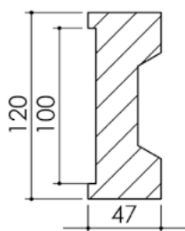
Montant côté articulation
