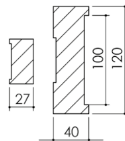
Montant côté battement en configuration 1 vantail
