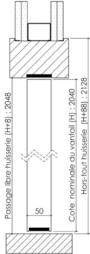
Montant côté articulation
