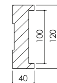
Montant côté battement en configuration 1 vantail
