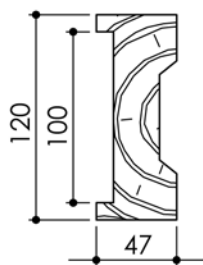
Montants
