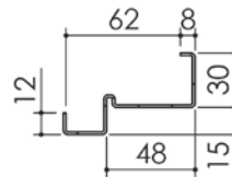
Huisserie isophonique
