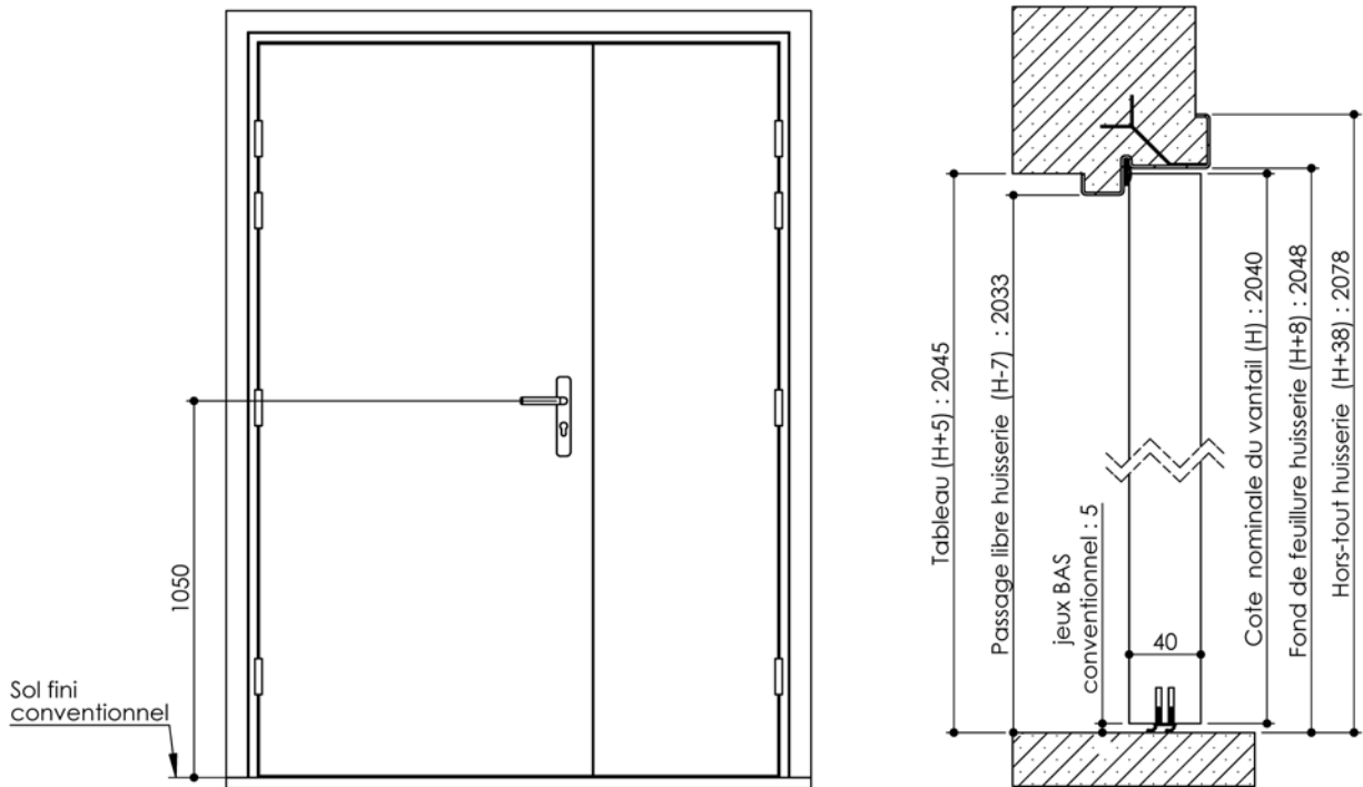
Huisserie isophonique
