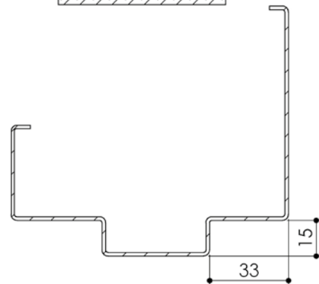
Huisserie non isophonique Pavillon 31
