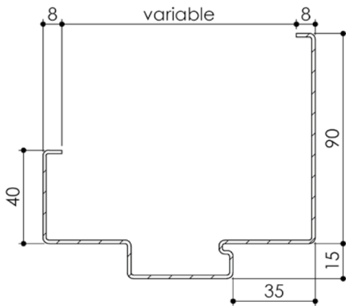
Huisserie isophonique Pavillon 31, 40
