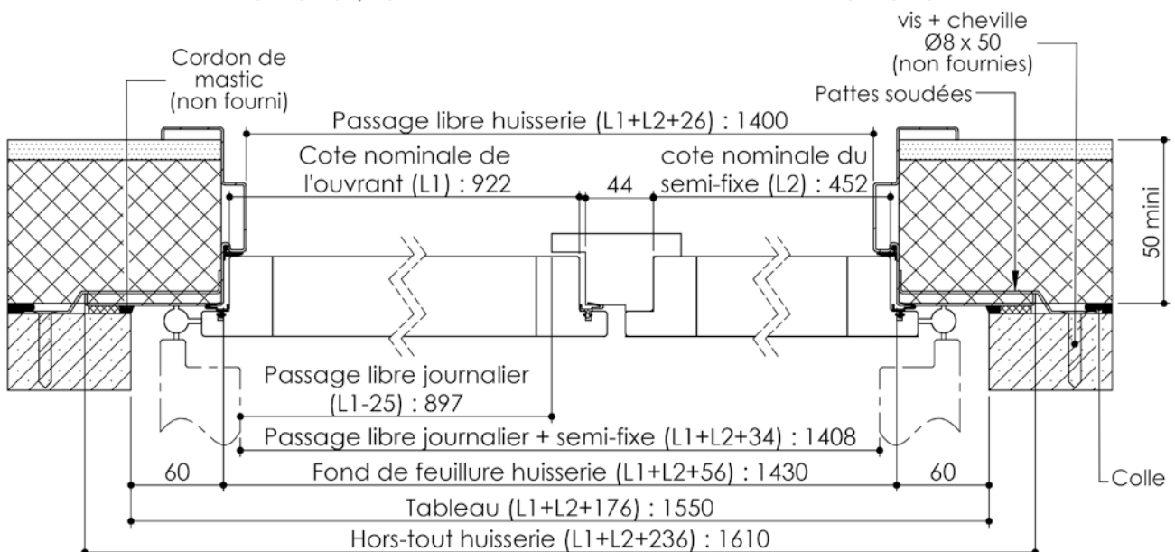
Huisserie isophonique Pavillon 31, 40
