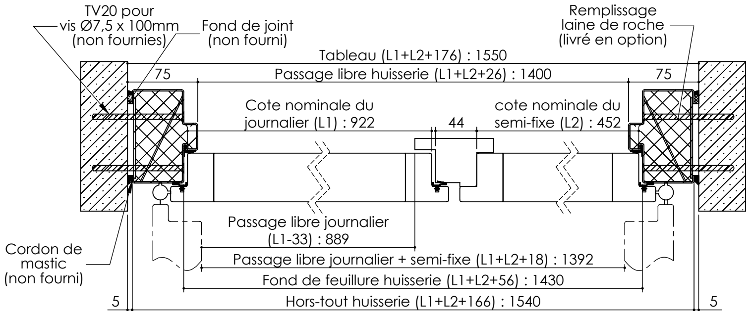
Huisserie isophonique Pavillon 31, 31 CR3, 40, 45, 45 CR3, MetalForce Villa BP1
