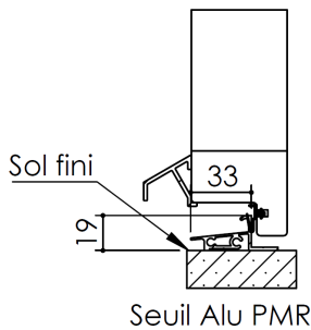
Détail bas de porte
