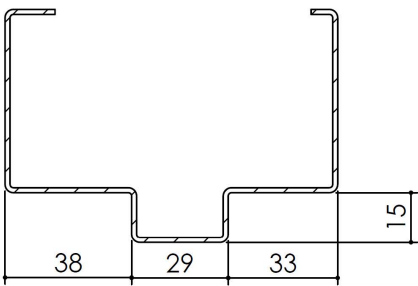
Huisserie non isophonique Pavillon 31, 31 CR3
