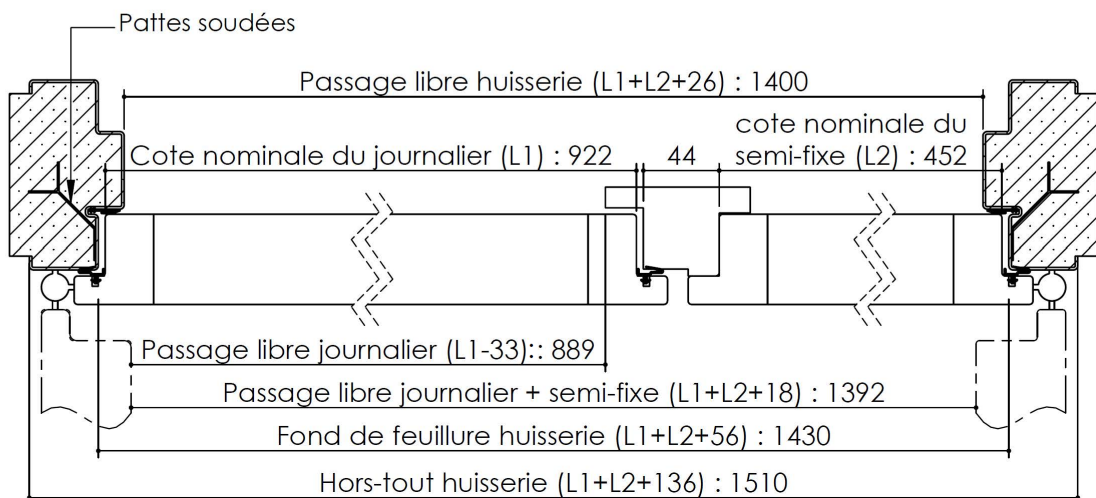
Huisserie isophonique Pavillon 31, 31 CR3 40, 45, 45 CR3, MetalForce Villa BP1
