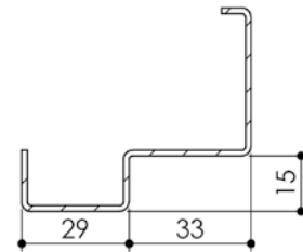
Huisserie non isophonique Pavillon 31, 31 CR3
