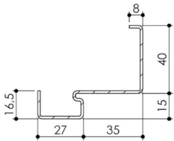
Huisserie isophonique Pavillon 31, 31 CR3, 40, 45 CR3, MetalForce Villa BP1
