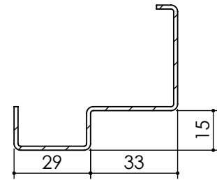
Huisserie non isophonique Pavillon service
